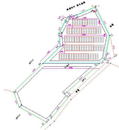
《太陽光パネル配置モデル図》
