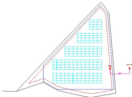
《太陽光パネル配置モデル図》
