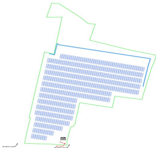
《太陽光パネル配置モデル図》
