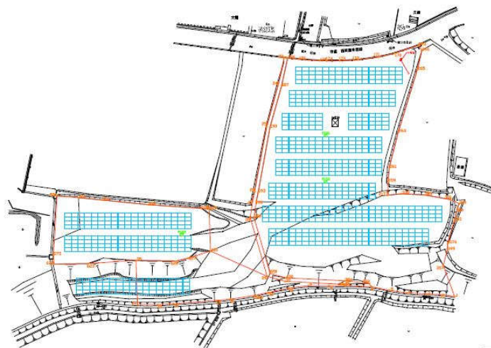
《太陽光パネル配置モデル図》
